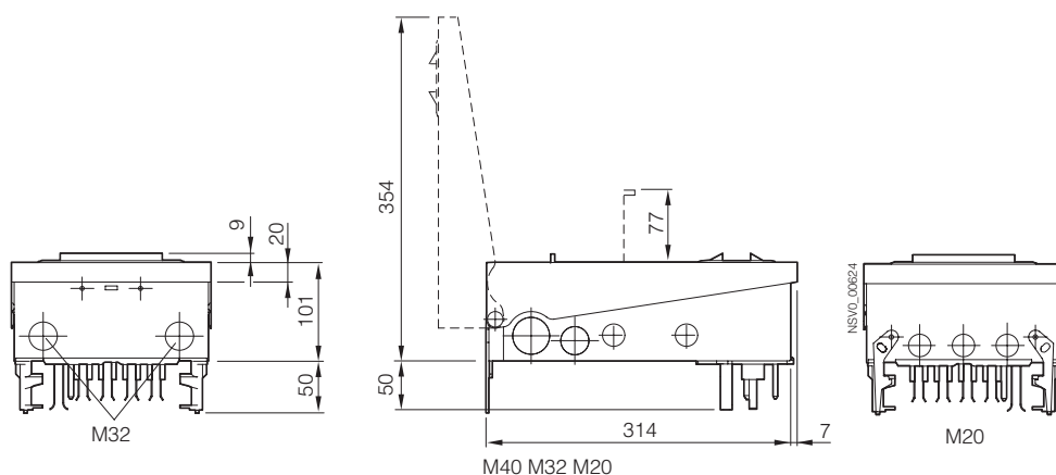
BD2-AK2X/F..., BD2-AK2X/GB..., BD2-AK2X/S...
