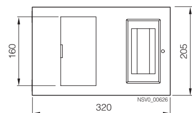
BD2-AK2M2/A...
