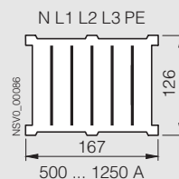
Секции шинпровода BD2A-3, BD2C-3, секции изменения направления, ввода питания BD2A-..., BD2C-...
