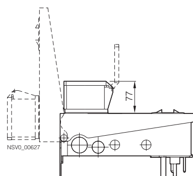
BD2-AK2X/CEE635S33 (/FORMP)
