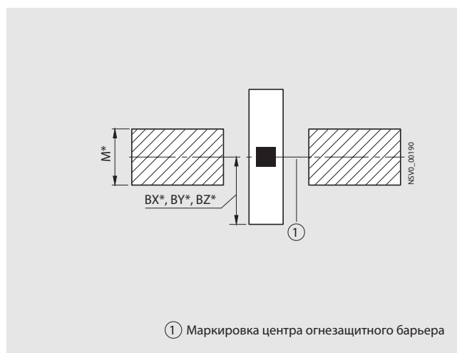
Положение в несгораемом перекрытии
