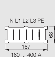
Секции шинпровода BD2A-3, BD2C-3, секции изменения направления, ввода питания BD2A-..., BD2C-...
