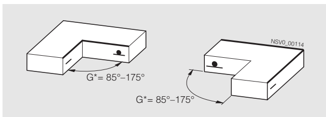
Слева: горизонтальная, вправо; BD2-...-LR-G*, BD2-...-LR-X*-G*, BD2-...-LR-Y*-G*, BD2-...-LR-X*/Y*-G* Справа: горизонтальная, влево; BD2-...-LL-G*, BD2-...-LL-X*-G*, BD2-...-LL-Y*-G*, BD2-...-LL-X*/Y*-G*
