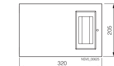
BD2-AK2M2/A...
