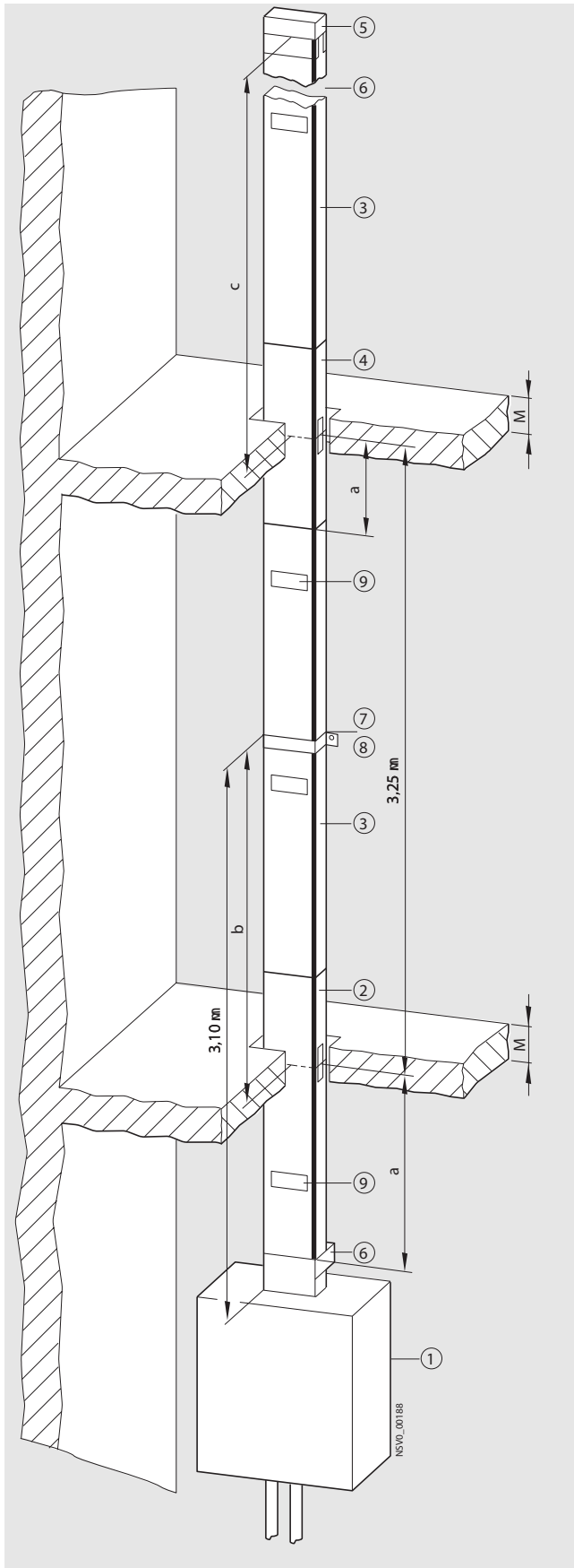
Схема установки
