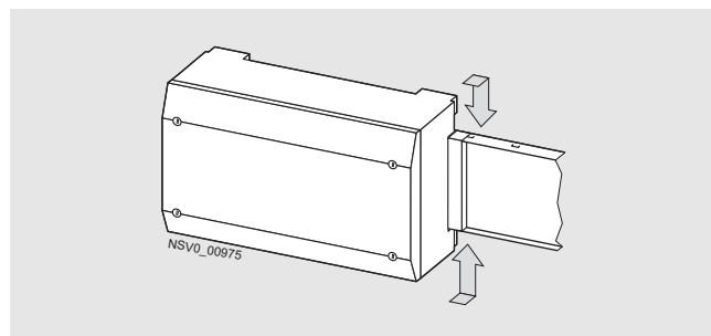
Боковая установка в конце участка шинпровода: BD01-KS
