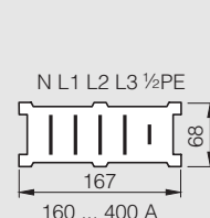
Секции шинпровода BD2A-2, BD2C-2
