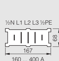
Секции шинпровода BD2A-1
